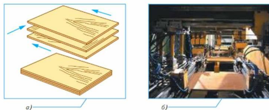
Рис. 5.5. Расположение направления волокон шпона в фанере (а) и производство древесно-стружечных плит (б)
