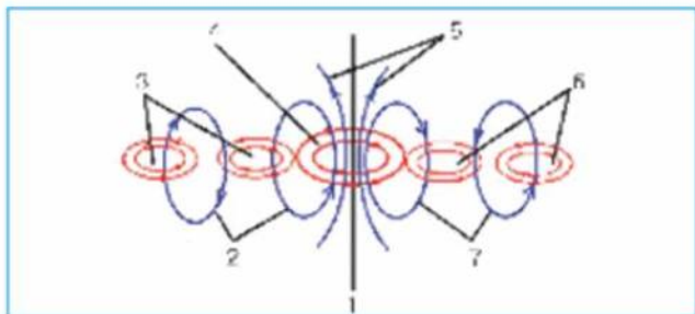
Рис. 8.12. Образование переменного распространяющегося электромагнитного поля: 1 — проводник; 2, 7 — новые магнитные поля; 3, 6 — новые электрические поля; 4 — переменное электрическое поле проводника; 5 — внешнее переменное магнитное поле
