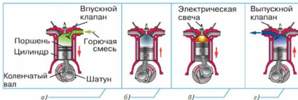
Рис. 4.11. Схема работы бензинового двигателя: а — всасывание воздуха; б — сжатие воздуха; в — впрыскивание топлива (рабочий ход); г — выпуск отработанных газов
