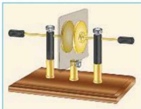
Рис. 8.4. Устройство конденсатора
